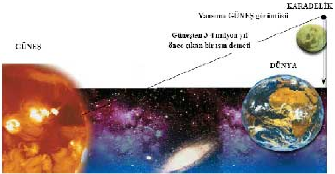
Şekil -4 İkinci olayın temsili resmi: Güneşten çıkan bir ısının bir Karadeliğten yansıması.
